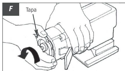
Contraiga el conjunto de rodillos
