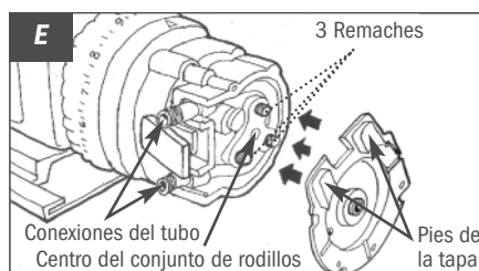
Alinee las aberturas de los tubos de la tapa cerca de las conexiones de los tubos
