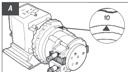
Modelos de caudal ajustable deben tener el anillo del caudal en 10
